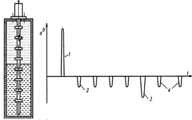
Рис. 2. Зонд с регулярными неоднородностями и его рефлектограмма [23]
