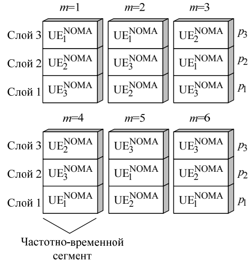
Рис. 2. Формирование комбинаций уплотнения
