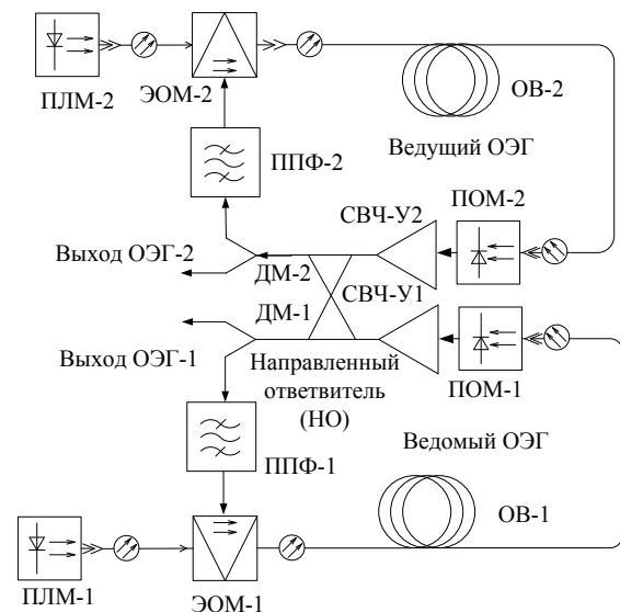
Рис. 3. Структурная схема ОЭГ с инъекционной синхронизацией мод
