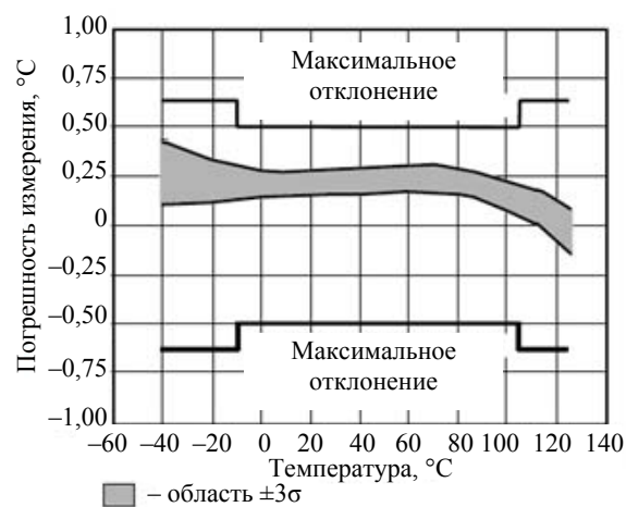
Рис. 2. Погрешность датчика температуры при напряжении питания 5 В
