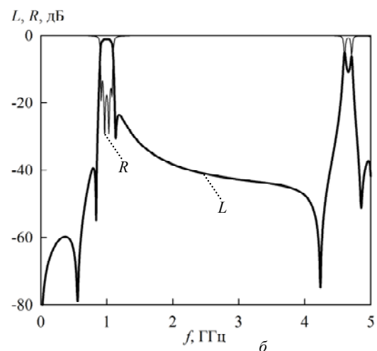
Рис. 2. АЧХ фильтра на основе 2D-электромагнитного кристалла в широком диапазоне частот (б) и в узком (а):
