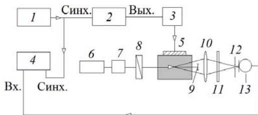
Рис. 3. Схема экспериментальной установки: 1 – генератор импульсов АК ИП-3301; 2 – ВЧ-генератор Agilent N5181B; 3 – ВЧ усилитель; 4 – осциллограф Tektronix TDS1012C-EDU; 5 – АО-затвор; 6 – лазер ЛГН 207А; 7 – коллиматор; 8 – поляризатор; 9 – непрозрачный экран; 10 – собирающая линза; 11 – светофильтр; 12 – пространственный фильтр; 13 – ФЭУ
