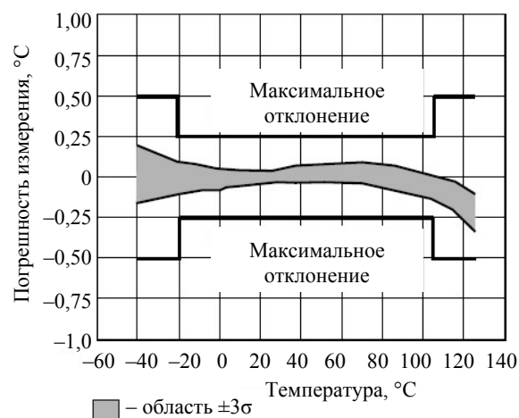
Рис. 3. Погрешность датчика температуры при напряжении питания 3,3 В
