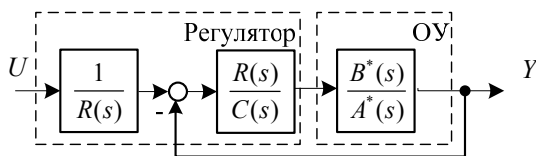
Рис. 3. Модель САУ с ПР
