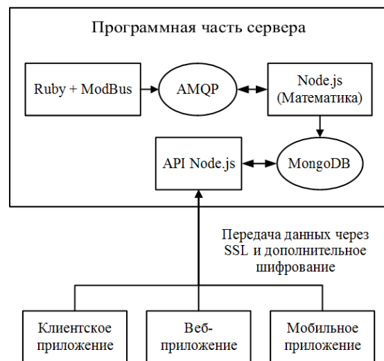
Рис. 2. Архитектура программной части системы
