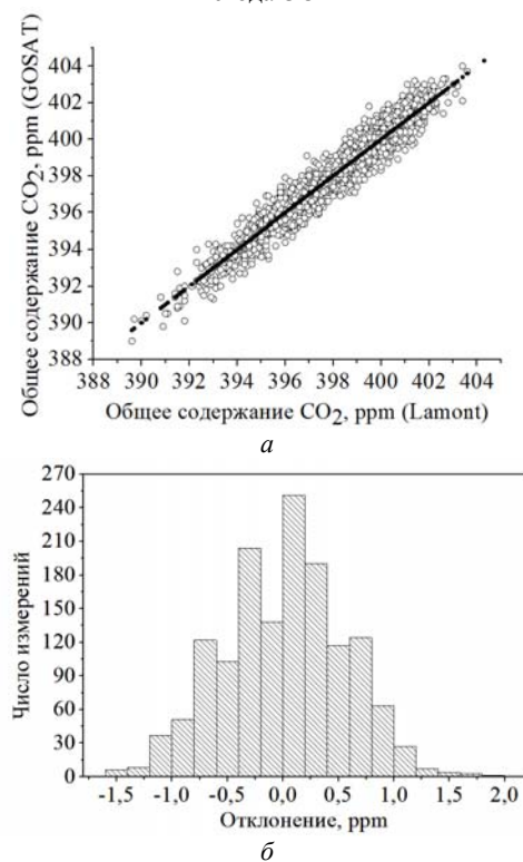
Рис. 3. Сравнение измеренных на станции TCCON Lamont и восстановленных общих содержаний CO 2 по данным спутникового прибора GOSAT (а) и отклонение этих значений друг от друга в виде гистограммы (б) для модифицированного метода ЭОФ
