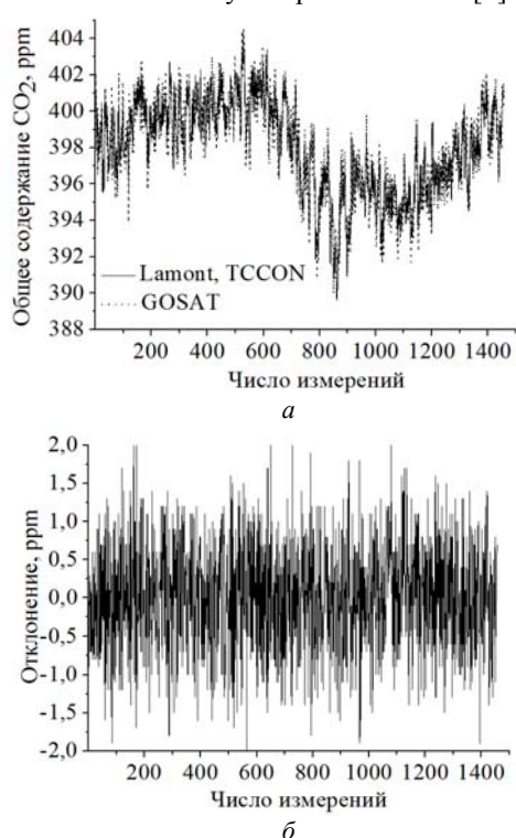
Рис. 1. Сравнение измеренных на станции TCCON Lamont и восстановленных общих содержаний CO 2 по данным спутникового прибора GOSAT (а) и отклонение этих значений друг от друга (б)
