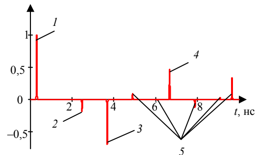
Рис. 4. Рефлектограмма измерительного зонда в многофазной среде
