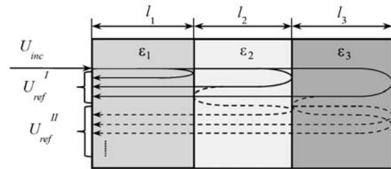
Рис. 3. Модель распространения сигналов
