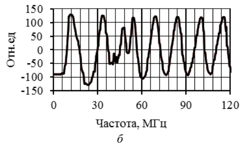
Рис. 4. Частотные характеристики КСВН пьезопреобразователя на основе: а – РКТР, б – ниобата лития
