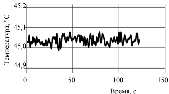
Рис. 6. Показания цифрового датчика в установившемся режиме
