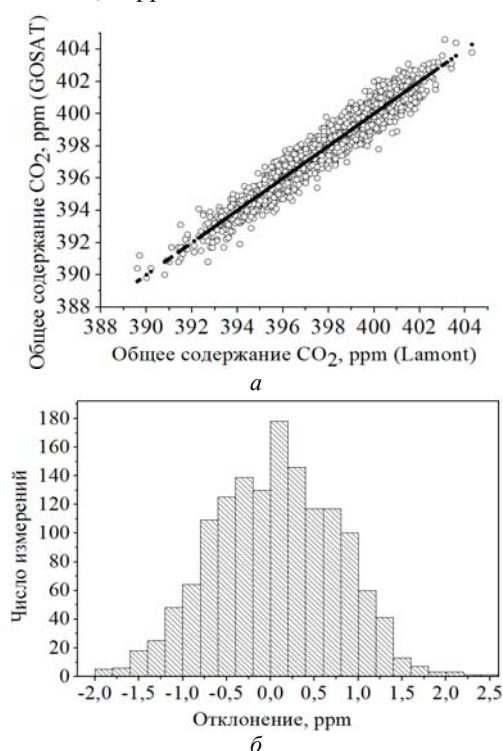
Рис. 2. Сравнение измеренных на станции TCCON Lamont и восстановленных общих содержаний CO 2 по данным спутникового прибора GOSAT (а) и отклонение этих значений друг от друга в виде гистограммы (б) для основного метода ЭОФ
