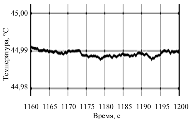
Рис. 5. Выходной сигнал САУ в установившемся режиме
