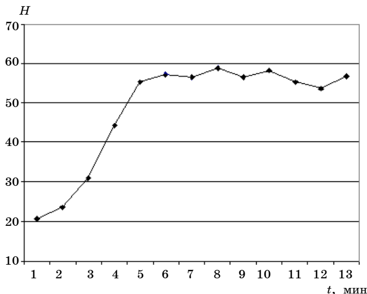
Рис. 1. Изменение энтропии IP-адресов назначения в передаваемых по сети пакетах с течением времени при распространении сетевого вируса
